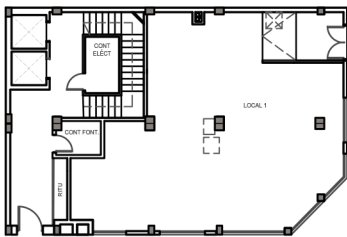
Planta baja Sup. construida 143.71 m²
